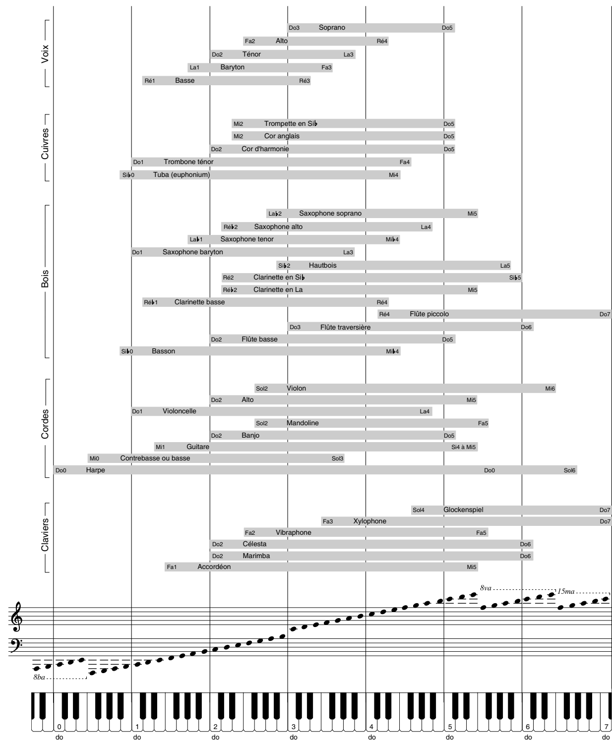
Fig. 68 Tableau de la tessiture des principaux instruments
